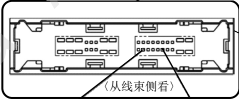
车辆 36 极连接器
